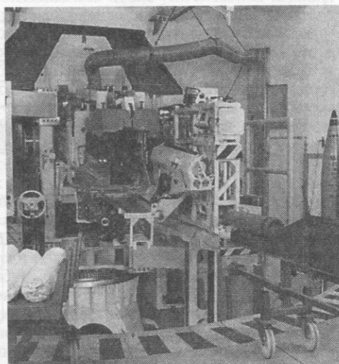
Рис. 2. Казенная часть пушки L52 с механизмом заряжания
