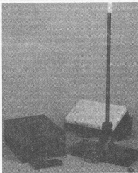
Рис. 4. Французский комплект аппаратуры опознавания, предназначенный для размещения на наземных объектах
